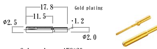
Crimp size : AWG#20 JMD-TK-201 (Y)
